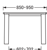
側面
