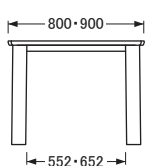
側面
